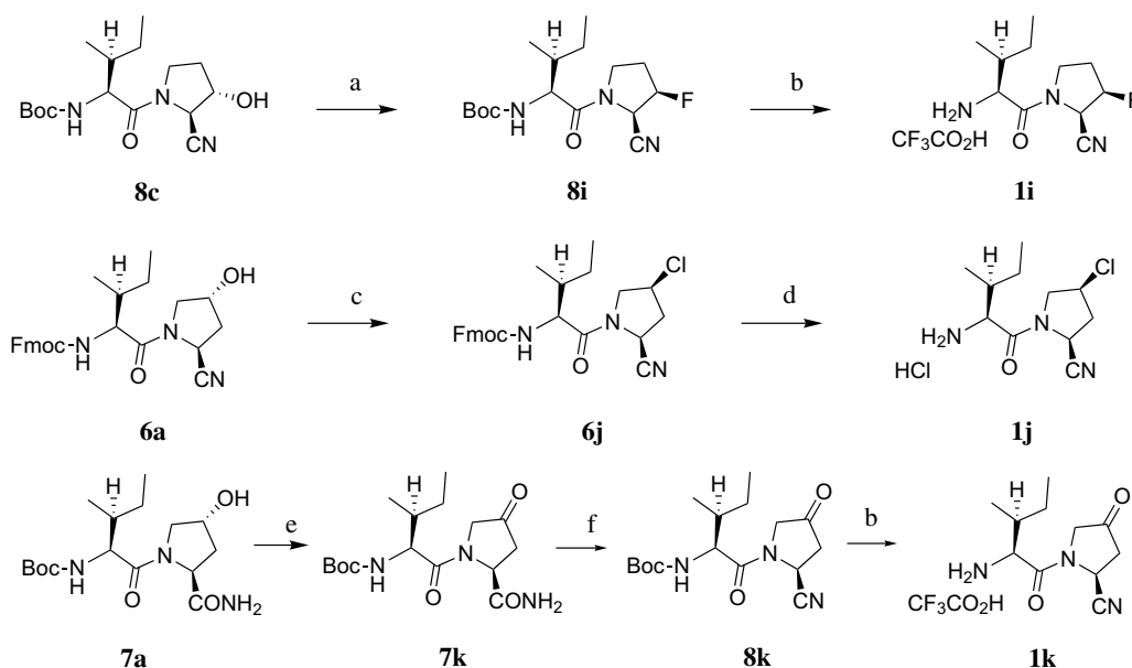
Scheme 2. Reagents: (a) DAST, CH 2 Cl 2 ; (b) TFA; (c) Ph 3 P, CCl 4 ; (d) Et 2 NH, 1,2-dichloroethane; then HCl; (e) PCC, MS4A, AcOH, CH 2 Cl 2 ; (f) (CF 3 CO) 2 O, N,N -diisopropylethylamine, THF.
